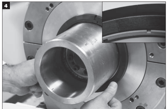
Nach Bedarf Kraft anwenden, um die Dichtung gleichmäßig in das Gehäuse zu pressen. Die Stöße zuerst in Richtung 6-Uhr-Stellung drücken.
