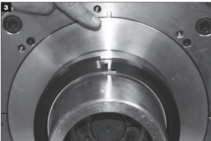
Die Bindegurte entfernen. Die geteilten Enden an der 12-Uhr-Position aufsuchen und miteinander verbinden. HINWEIS: Nach Abschluss des Einbaus ist eine Lücke zwischen den geteilten Enden des Dichtrings zulässig.
