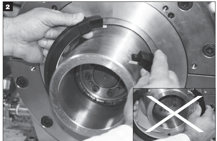
Die Dichtung an den zwei Bindegurten halten und die Dichtung um die Welle wickeln.
